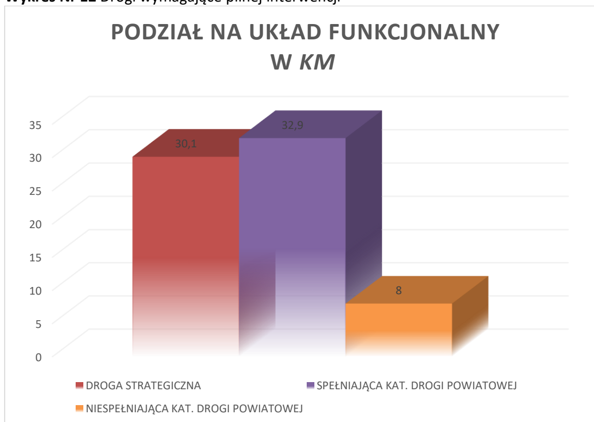
Wykres Nr 12 Drogi wymagające pilnej interwencji
